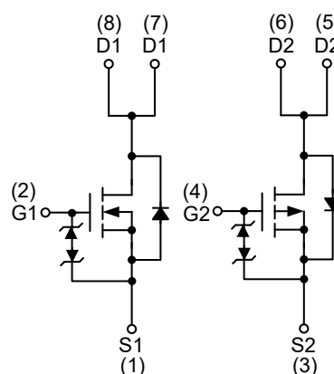
N-Channel MOSFET P-Channel MOSFET
