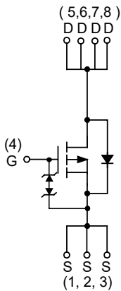
P-Channel MOSFET
