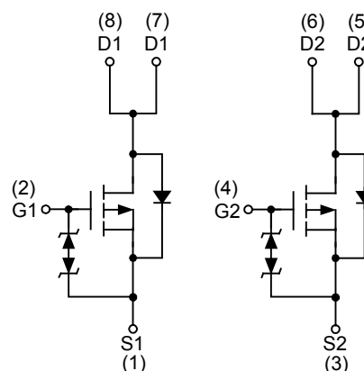
P-Channel MOSFET
