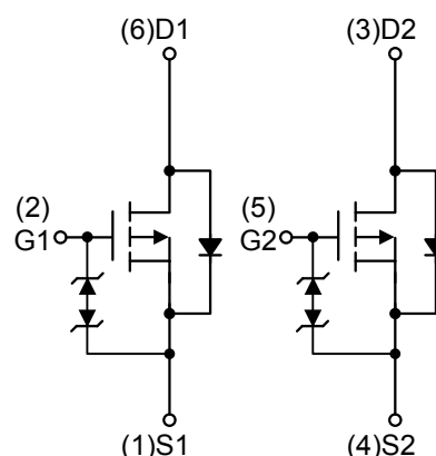
P-Channel MOSFET
